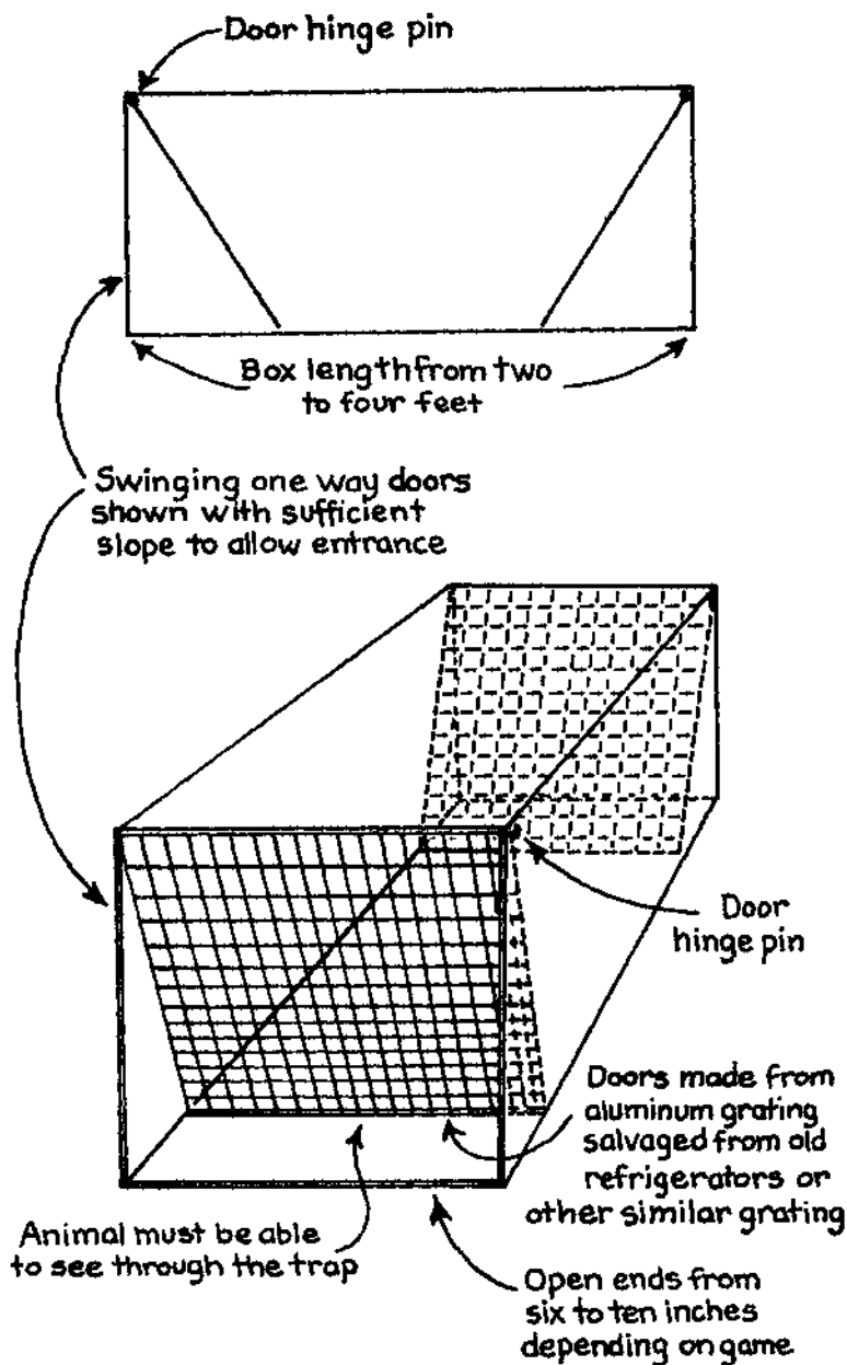
PUSH DOOR BOX TRAP
